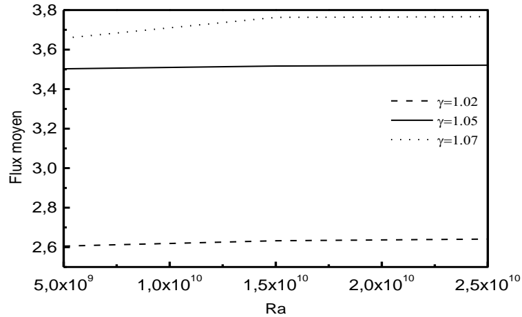
Fig.5: Effet de \gamma sur le transfert de chaleur global à travers le bâtiment.
