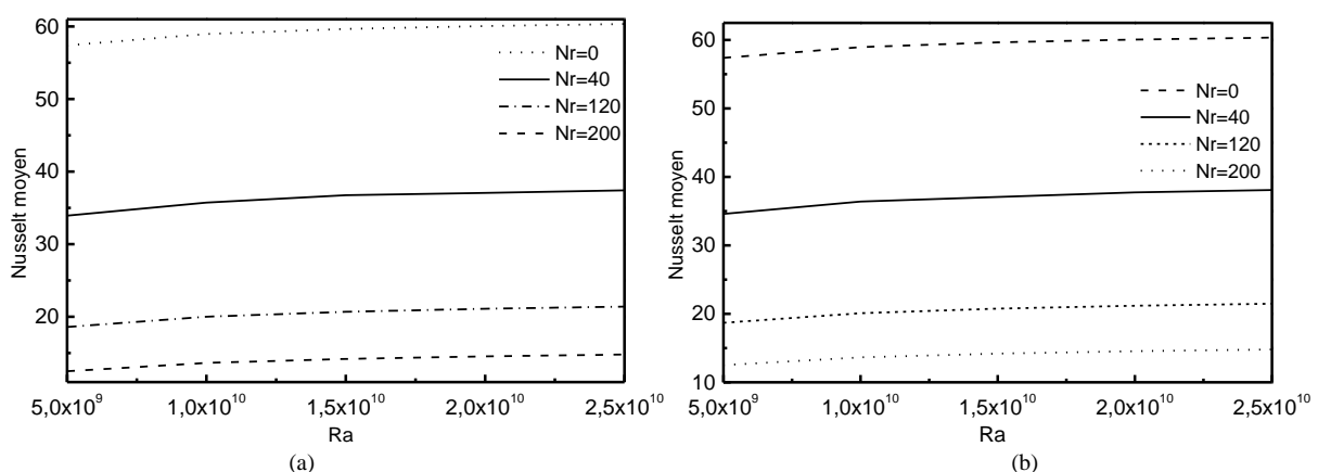
Fig.2: Effet de Nr sur la convection naturelle : (a) sur la surface intérieure gauche; (b) sur la surface intérieure droite.
