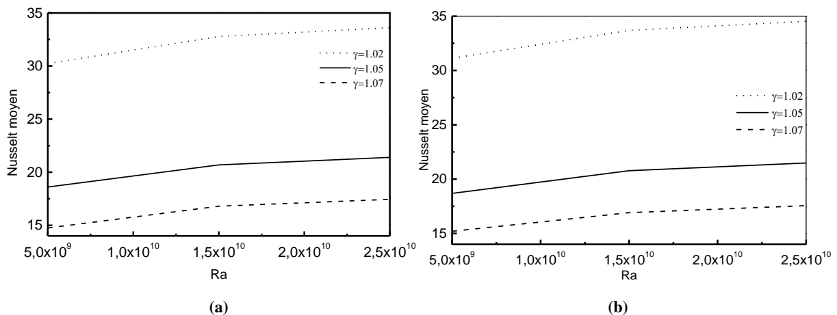
Fig.4: Effet de \gamma sur la convection naturelle : (a) sur la surface intérieure gauche; (b) sur la surface intérieure droite.
