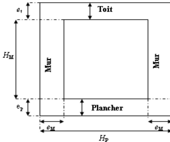
Fig.1: Configuration du bâtiment étudié.
